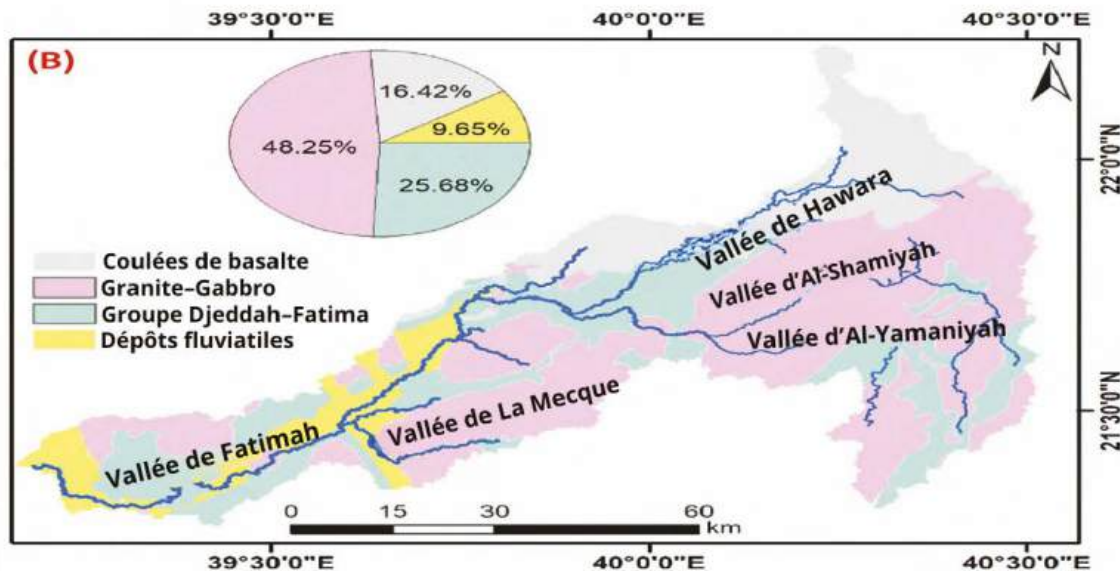
La figure supérieure (A) présente une carte géologique de la vallée de Fatimah, indiquant les unités rocheuses et les bassins d'écoulement. La figure inférieure (B) illustre la classification des proportions de roches et de sédiments de la vallée (modifiée d'après Abdelkareem et al., 2023).
