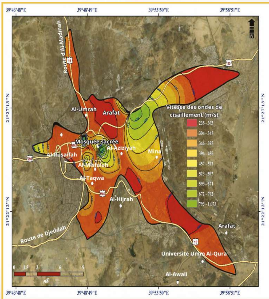
Carte de répartition de la vitesse des ondes de cisaillement dans la ville de La Mecque jusqu'à une profondeur de 30 m
