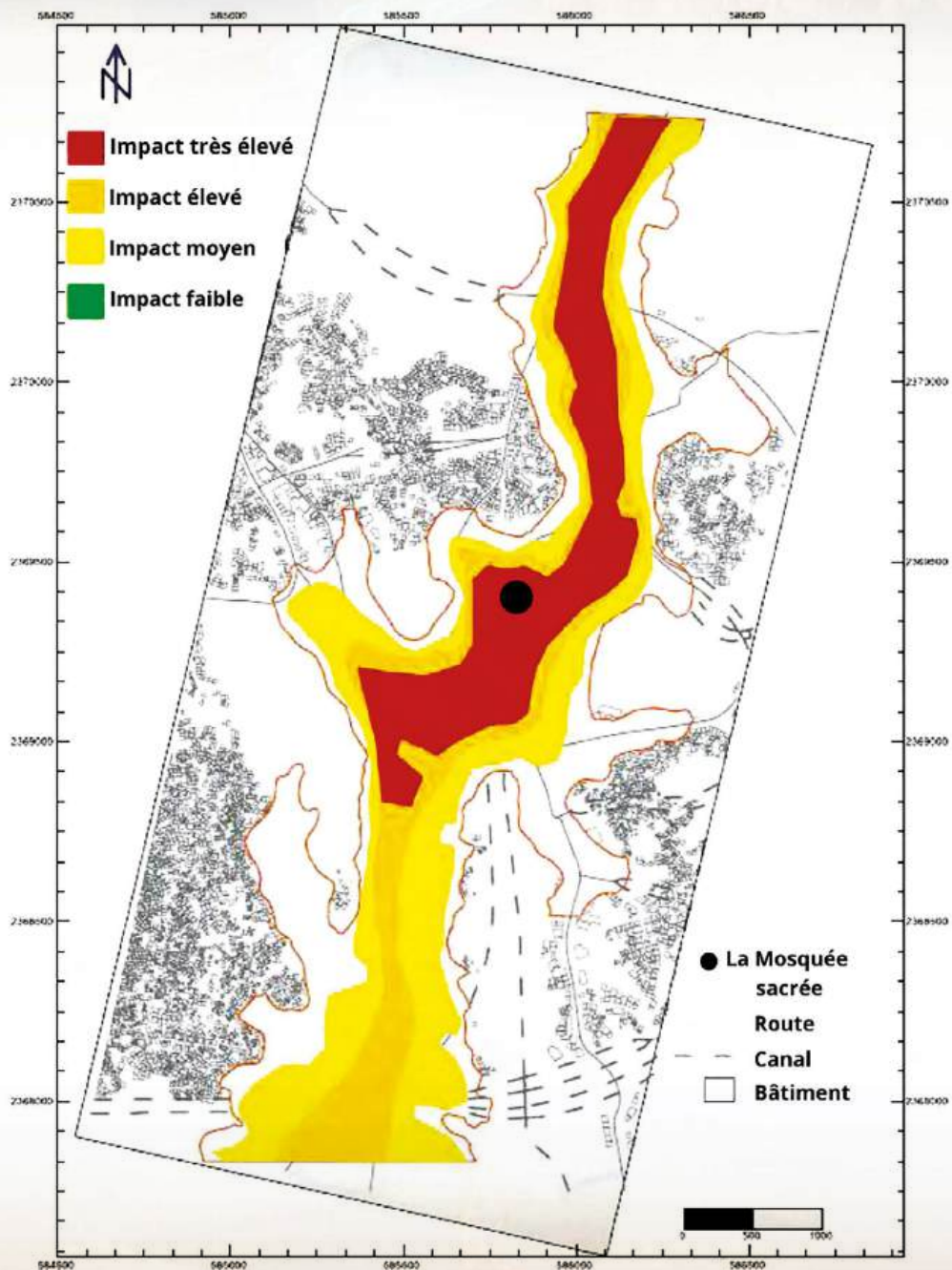
Carte illustrant l'impact des bâtiments de grande hauteur et des fondations sur le niveau d'eau du puits de ZamZam (modifiée à partir de Salam, 2015)
